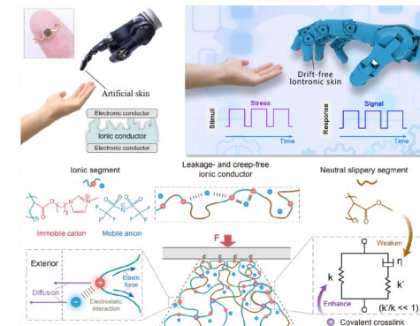
超弹性聚电解质离子导体的力学设计及其可计量柔性压力传感 (Nat. Mater., 23: 1107, 2024)
