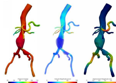
基于医学影像的腹主动脉瘤血液 -血管耦合建模 (Comput. Methods Appl. Mech. Engrg., 394: 114852, 2022)
