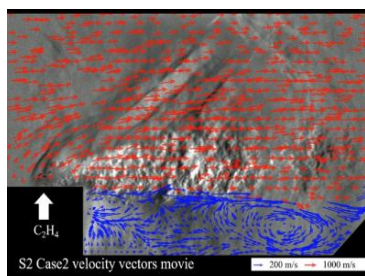
超声速燃烧冲压发动机中 的高时空分辨流场 (Combust. Flame, 269: 113705, 2024)
