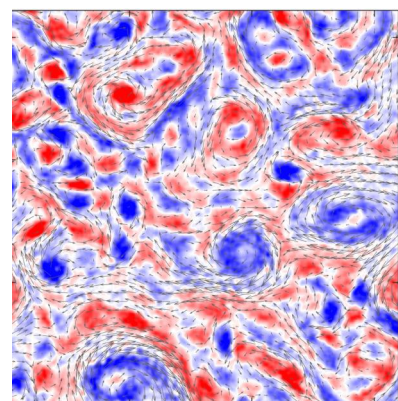
准二维湍流中的多尺度涡结构 (Phys. Rev. Lett. 130: 214001, 2023; J. Fluid Mech., 996: A39, 2024)
