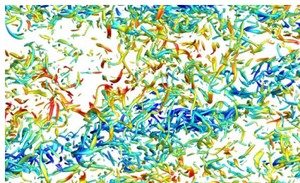
可压缩混合层中大尺度 对小尺度结构的调制效应 (J. Fluid Mech., 947: A38, 2022)
