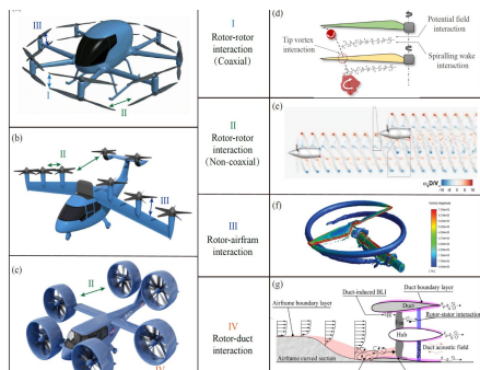
典型eVTOL飞行器构型及 其主要噪声源机制 (Prog. Aerosp. Sci., 161: 101184, 2026)
