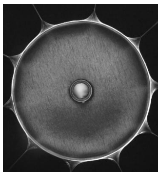
在指甲盖大小的圆片上 实现了上千个泰勒锥 (Phys. Rev. Lett. 126: 064502, 2021)
