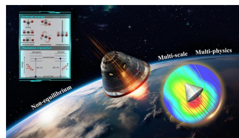
辐射气体动力学的动理论建模和多尺度计算 (J. Fluid Mech., 965: A13, 2023)
